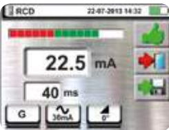
Risultato test a rampa su RCD.
